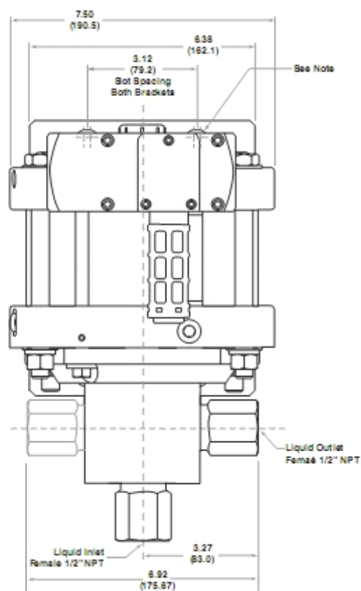
前视图
