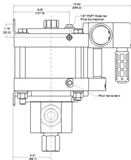
左视图
