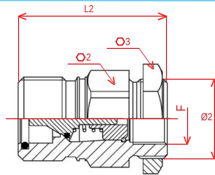
coupleur mâle / plug
