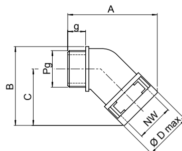
Dimensions Dimensionen
