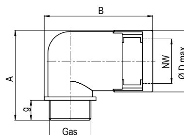
Dimensions Dimensionen
